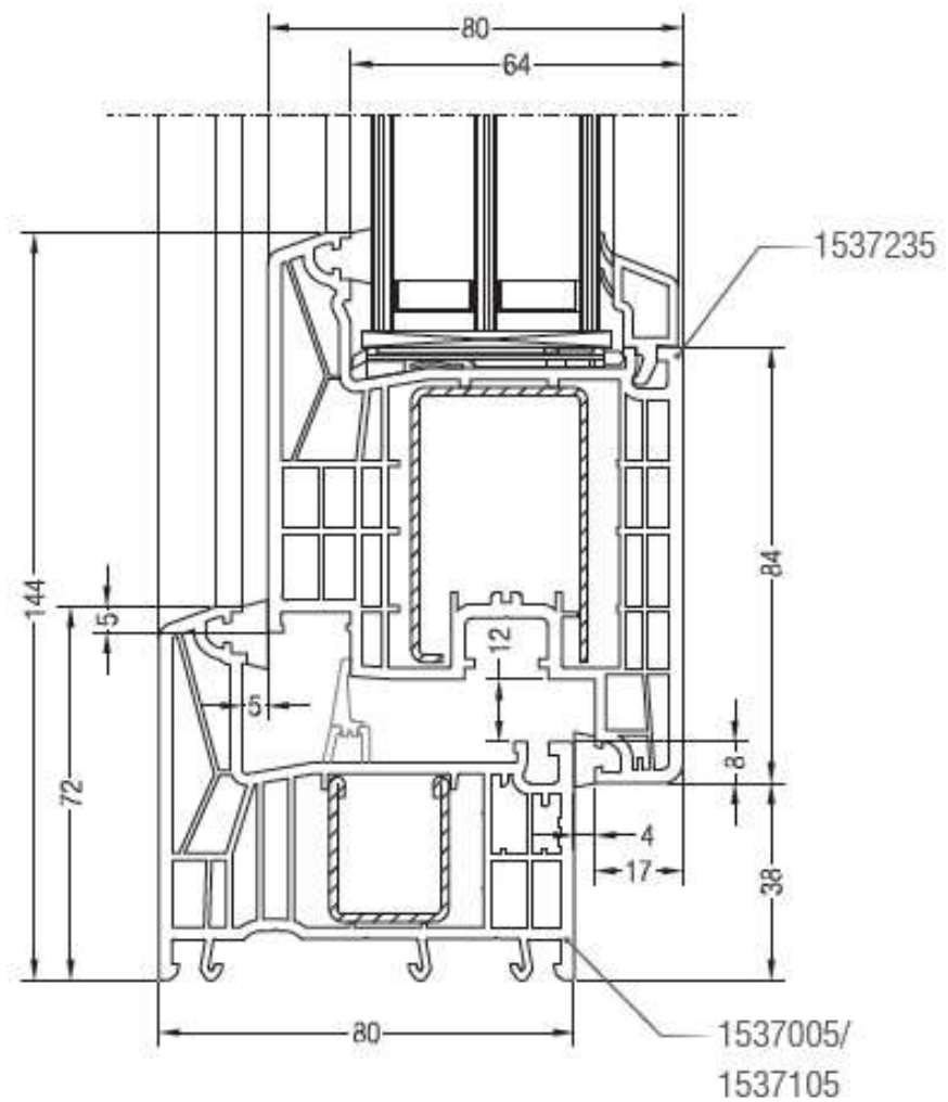
Sezione nodo anta dritta da 84 mm
