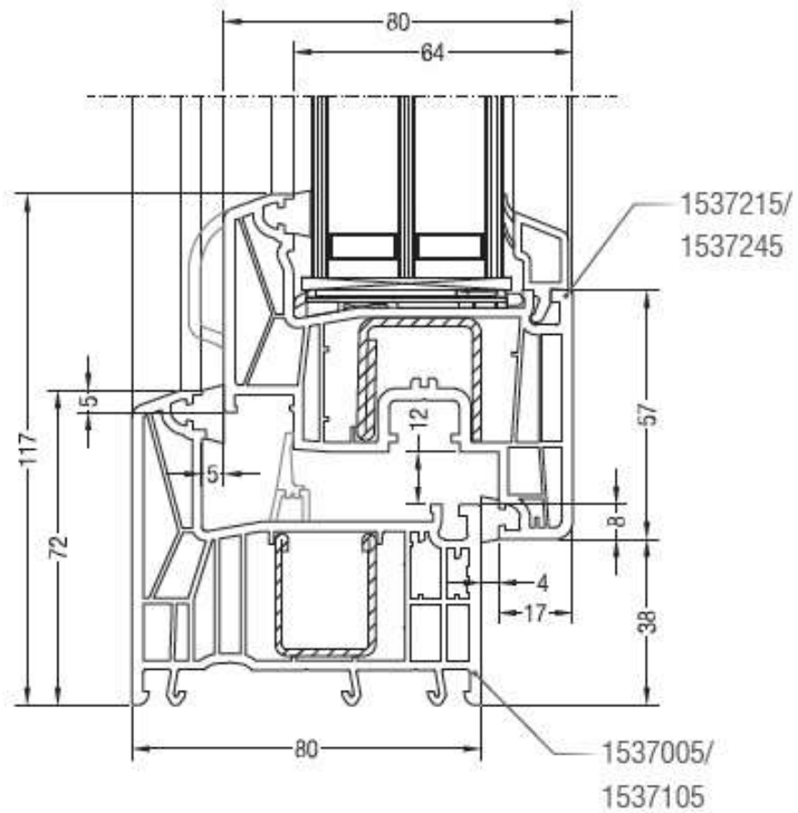
Sezione nodo anta arrotondata/dritta da 57 mm
